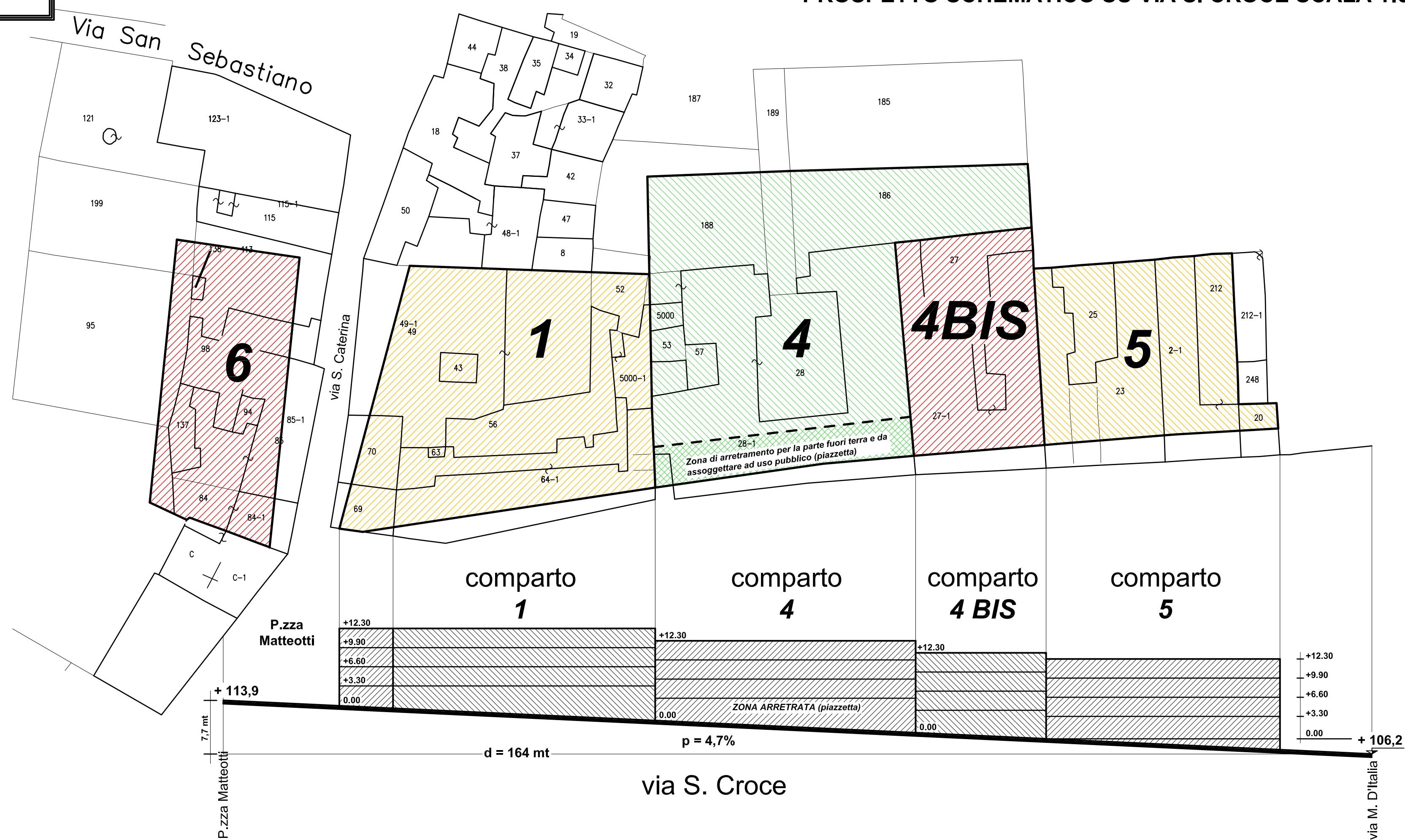
PROSPETTO SCHEMATICO SU VIA S. CROCE SCALA 1:500
